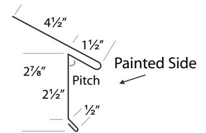
DRIP EDGE
