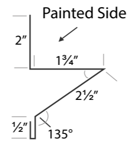
HR BASEGUARD
