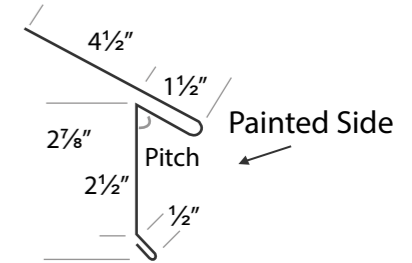
BULLNOSE DRIP EDGE
